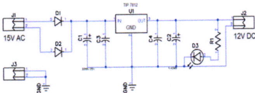
Gambar 7. Skema Power Supply 12 Volt
