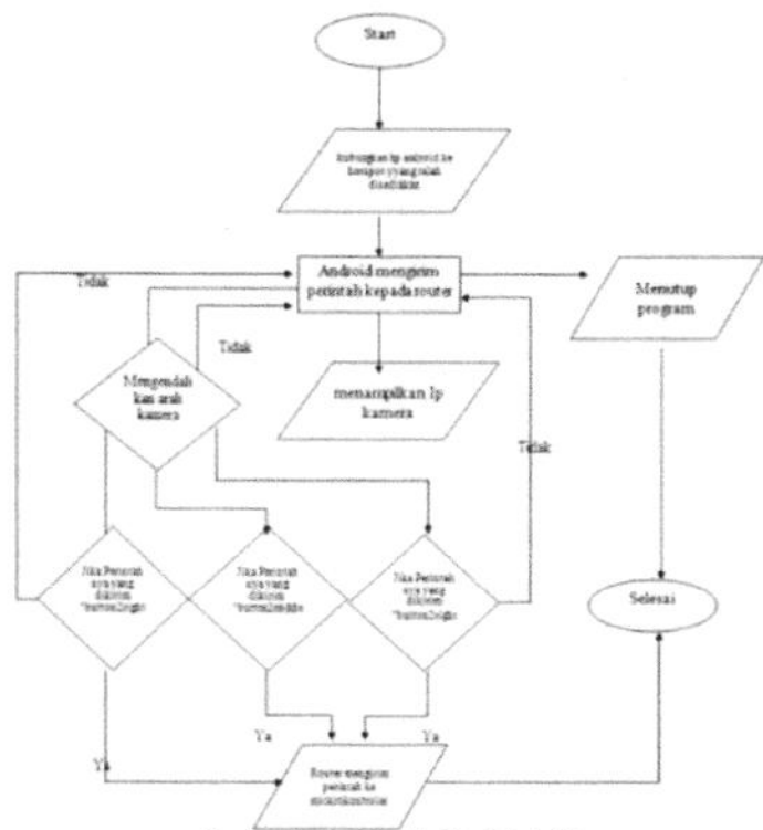
Gambar 2. Flowchart Aplikasi Android
