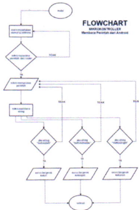
Gambar 3. Flowchart mikrokontroler
