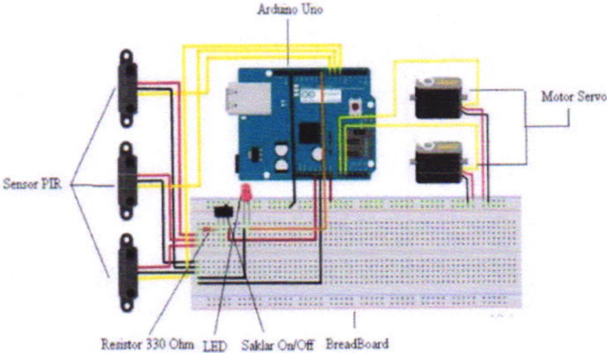
Gambar 5. Rangkaian Alat
